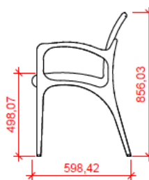
4 LATERAL - ITEM 43 1 : 25
