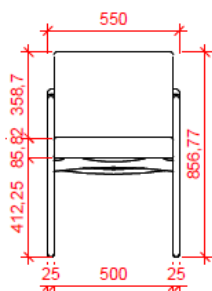
3 FRONTAL - ITEM 43 1 : 25
